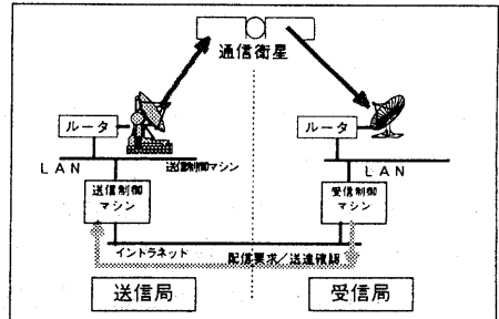
図1 衛星利用共有型情報配信システムの構成
