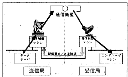
図2 アプリケーションの構成
