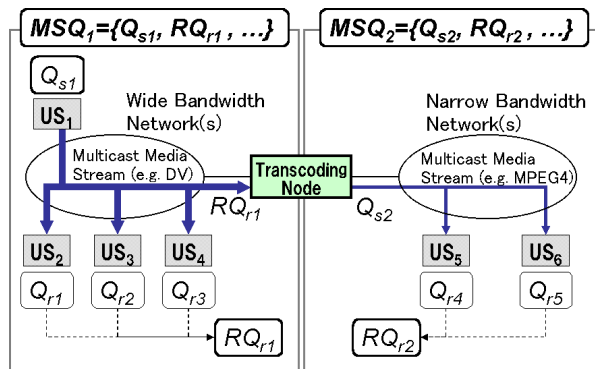
図 6: トランスコーディングノードと MSQ
