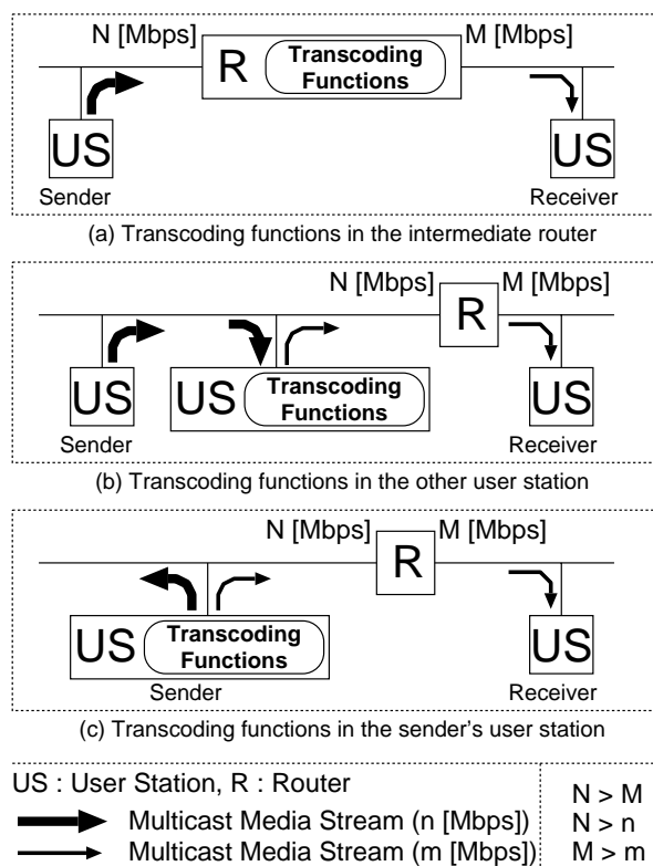
図 2: トランスコーディング ノード
