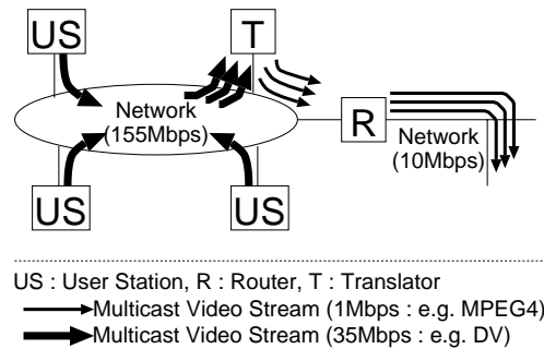
図 1: トランスレータ
