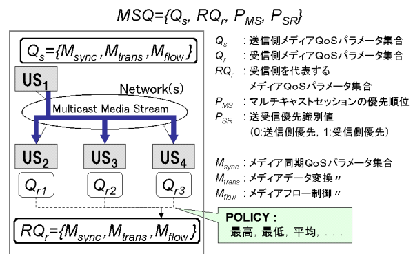
図 5: マルチキャストセッション QoS パラメータ集合
