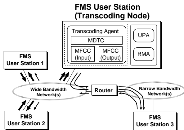
図 4: トランスコーディングエージェント
