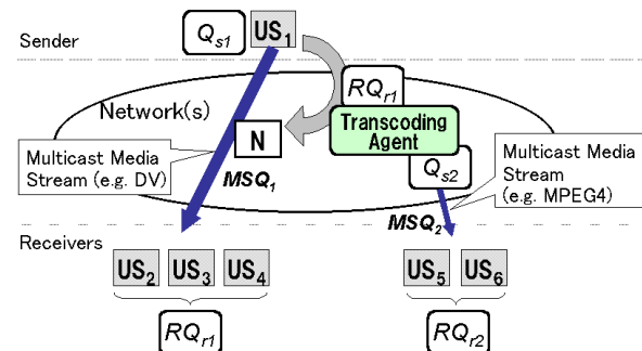
図 7: トランスコーディングノードの動的な配置
