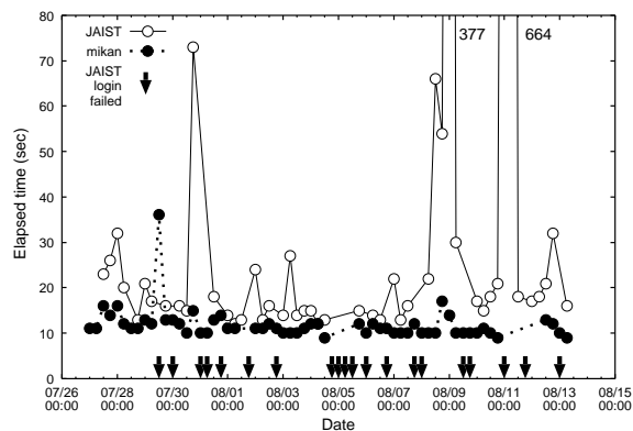
図 5: FTP サーバから直接取得した場合と「みかん」を経由した場合のファイル取得時間
