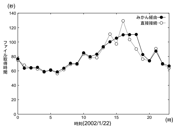
図 2: ATR からのファイル取得時間
