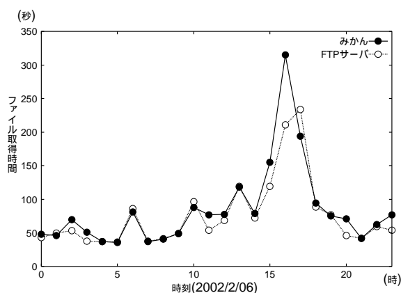
図 3: JAIST からのファイル取得時間
