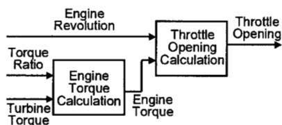
図2 制御ブロック図の例
