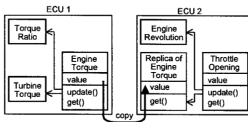
図4 時間駆動分散オブジェクトモデルの例
