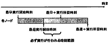
図 4 ノードのスケジューリング可能時刻範囲
