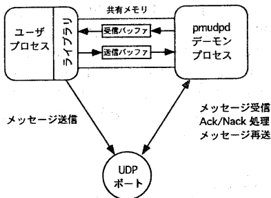
図2 PM/UDP の構成
