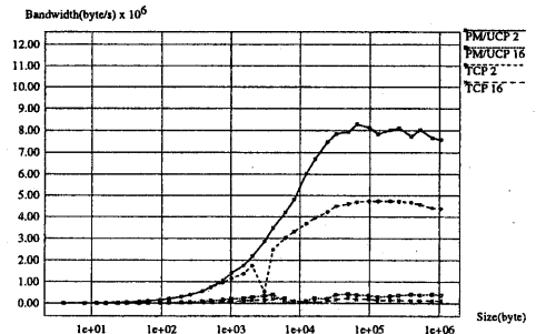
図7 MPI: Alltoall
