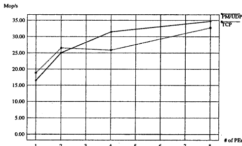
図 8 NPB2.3: CG (Class S)
