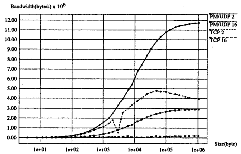
図6 MPI: Allgather
