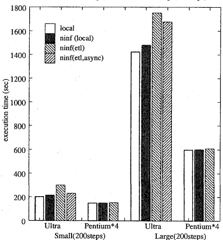
図6 netCFDの性能
