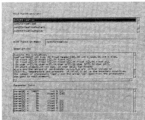
図1 NinfBrowser
