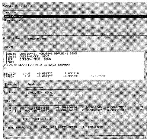
図4 netMO GUI
