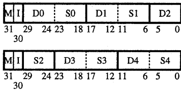
図 2: BISC-2 の命令形式
