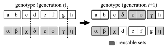
図 6 共通遺伝子の局所性と再利用可能性
