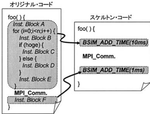
図2 プログラム・コードの抽象化
