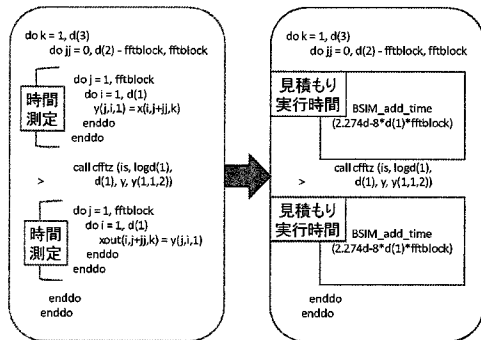
図 4 レベル 3 での FFT コード抽象化
