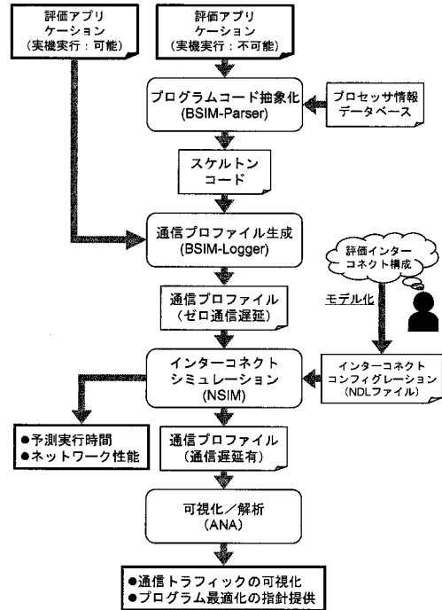
図 1 システム性能評価環境 PSI-SIM のワークフロー
