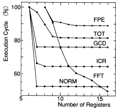
図 8: レジスタ数と実行サイクル数の関係
