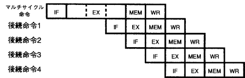
図 6: マルチサイクル命令の制御
