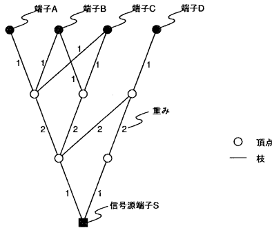
図 7: MPFA による配線処理 (1)
