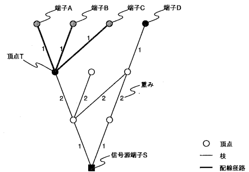
図 9: MPFA による配線処理 (3)
