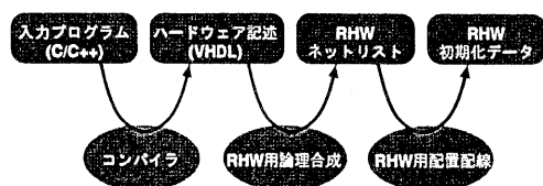
図 4: RHW1 におけるマッピングの流れ
