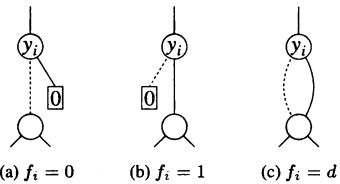
図1 不完全定義関数を表現するBDD_for_CF
