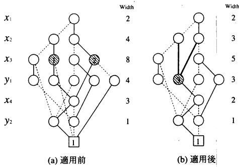
図5 アルゴリズム1を適用した BDD_for_CF
