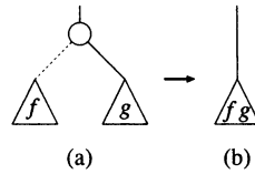
図 4 文献[12]の簡単化法
