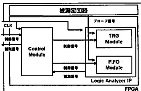
図6 ロジックアナライザ IP のブロック図
