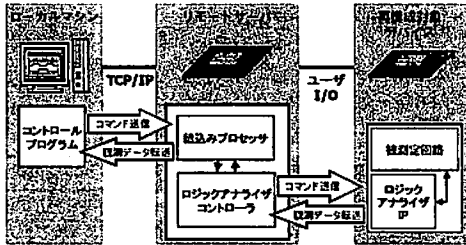
図 3 信号観測環境
