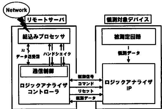
図 5 遠隔地側のリモートサーバと観測対象デバイスのブロック図
