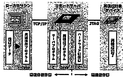
図 1 遠隔再構成環境
