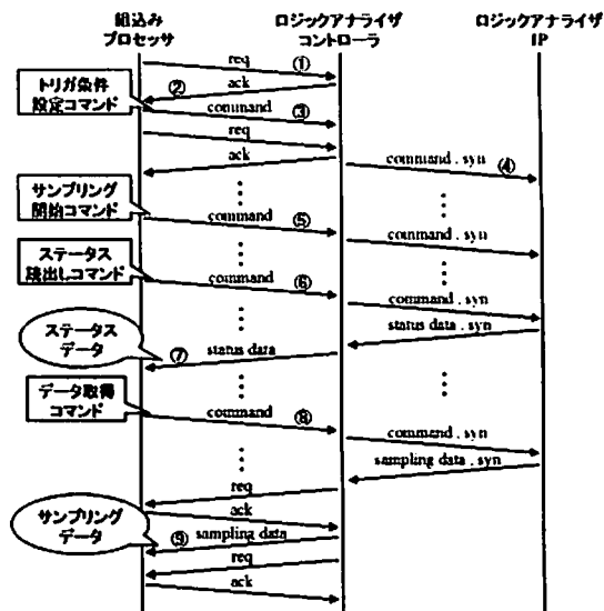
図7 通信フロー図
