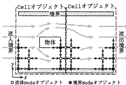
図 1: 数値風洞と計算領域分割の概念図
