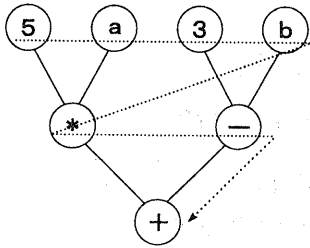
図 1: 式 (5*a)+(3-b) の構文木
