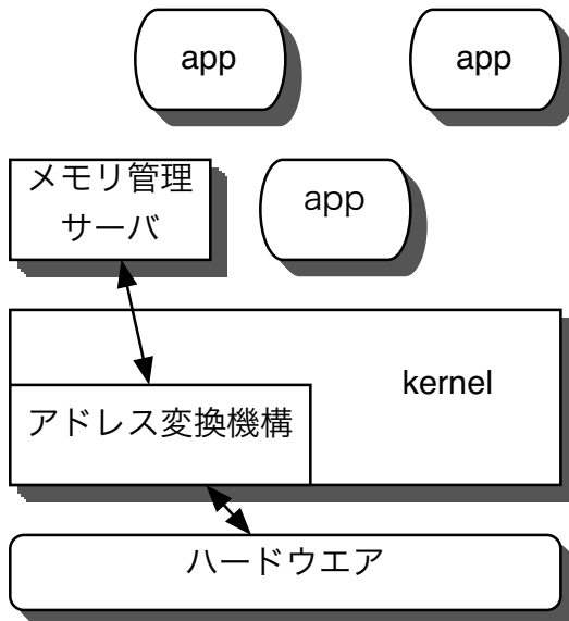
図 1: Lambda のメモリ管理機構の構成
