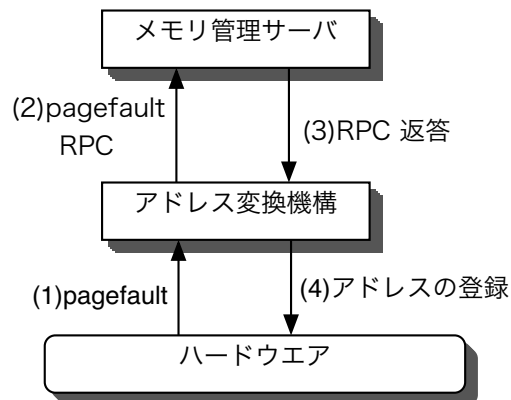
図 2: ページフォルトハンドリング
