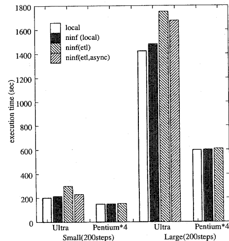
図6 netCFDの性能
