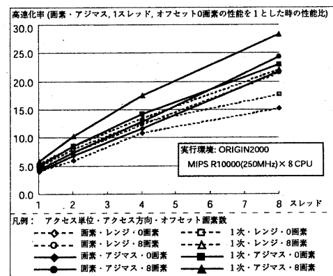
図11 アクセス方法と実行性能
