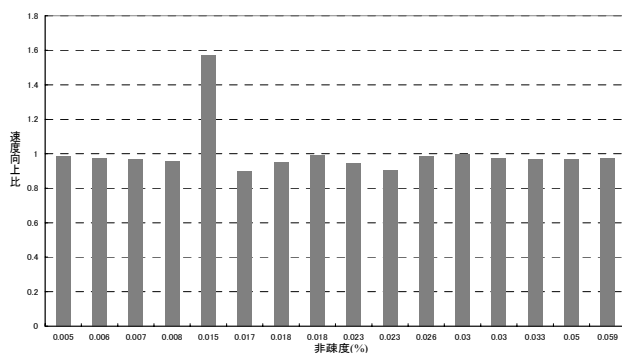
図 6 デフォルト OP に対する SLU' の速度向上比 (非疎度 0.005~0.059)
