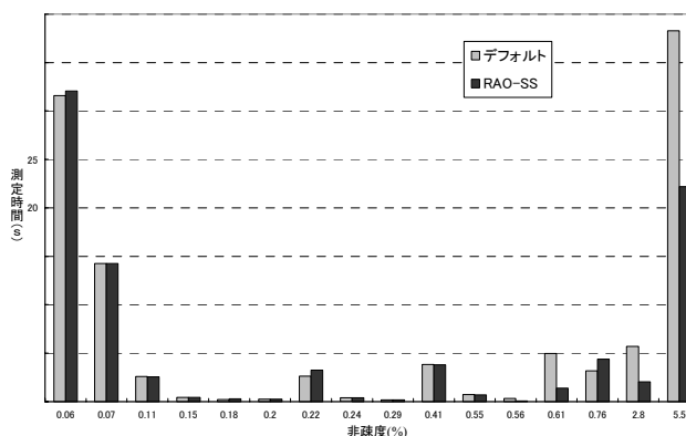
図 9 RAO-SS とデフォルトの実行時間 (非疎度 0.060~5.5)
