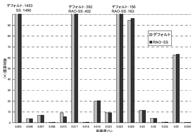
図 8 RAO-SS とデフォルトの実行時間 (非疎度 0.005~0.059)
