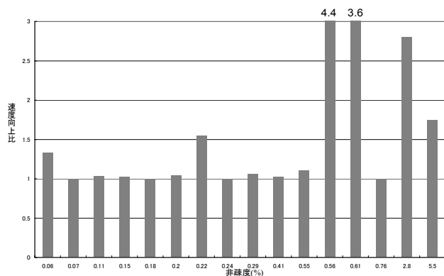
図 5 デフォルト OP に対する最適 OP の速度向上比 (非疎度 0.060~5.5)
