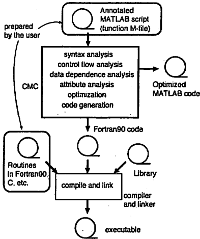
図2 CMCによるプログラム解析とコード出力の流れ
