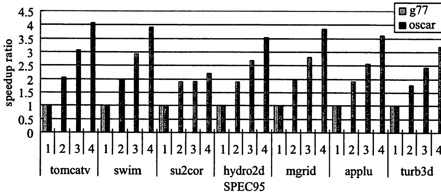
図8 MPCore 上での速度向上率
