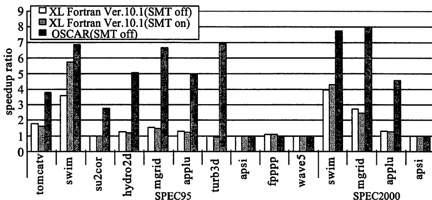
図 6 p5 550Q 上での速度向上率
