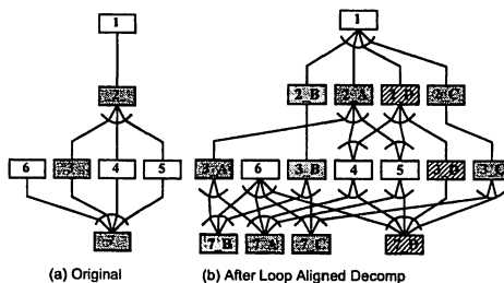
図4 粗粒度タスク間キャッシュ最適化
