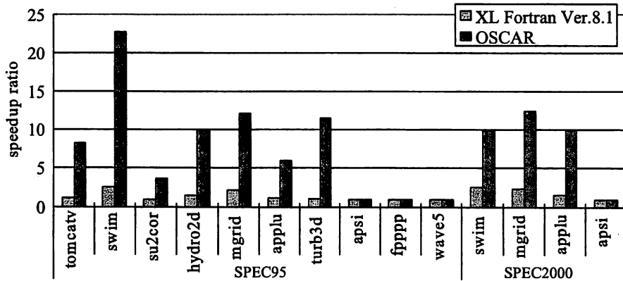
図7 pSeries690 上での速度向上率
