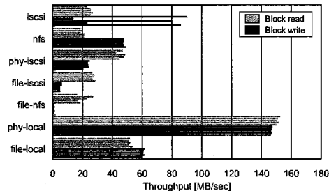
図 4 ドメイン U での Sequential I/O の性能
