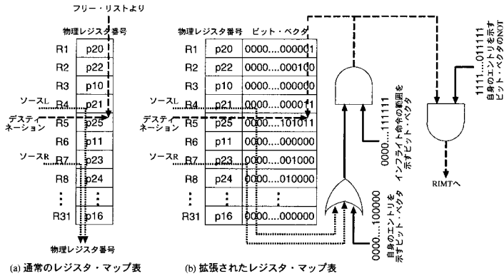
図 3 レジスタ・マップ表の拡張
