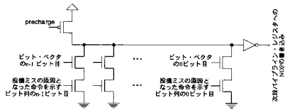
図7 パイプライン中のビット・ベクタと無効化対象を示すビット列の比較器
