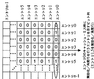
図 4 再発行行列表 (RIMT)
