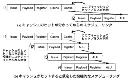
図2 命令発行レイテンシの長いプロセッサにおけるロード命令に依存する命令のスケジューリング
