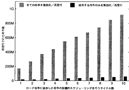
図10 投機的スケジューリングを行うサイクル数と再発行される命令数 (SPEint2000)
