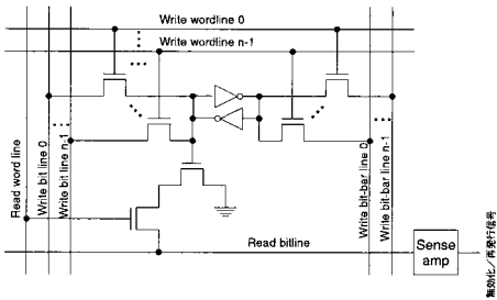
図6 RIMTの1bitセルの構成
