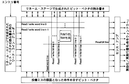
図5 RIMTの内部構造の概要
