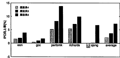
図 5 CB-BTP の IPC 向上率
