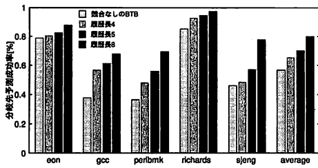
図 6 ハイブリッド予測器の予測精度
