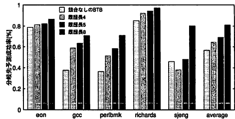
図 4 CB-BTP の予測成功率
