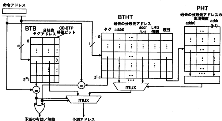
図3 BTBとCB-BTPのハイブリッド構成
