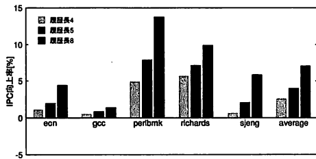
図 7 ハイブリッド予測器の IPC 向上率
