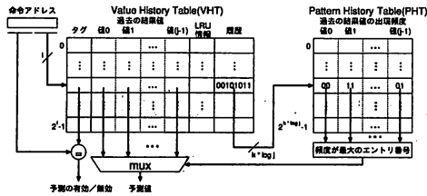
図1 コンテキスト・ベース値予測器(予測時の動作)
