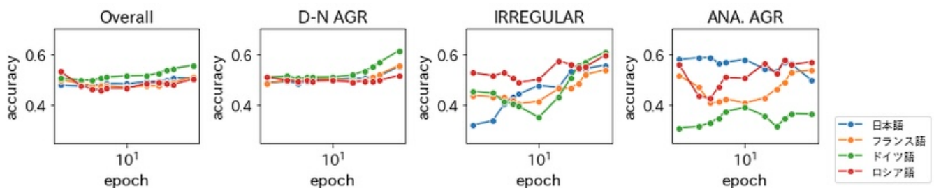
図 2: 第二言語学習中の各エポックにおける文法能力の評価結果 (抜粋)
