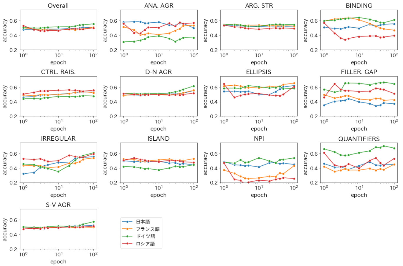
図 A.1: 第二言語学習中の各エポックにおける文法能力評価
