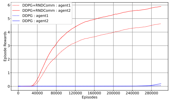
図 2: RNDComm (赤線) と DDPG のみ (青線) の学習過程の比較
