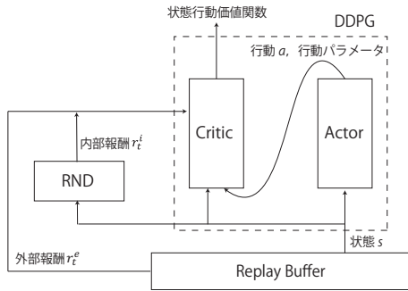
図 1: RND と DDPG を組み合わせたモデル
