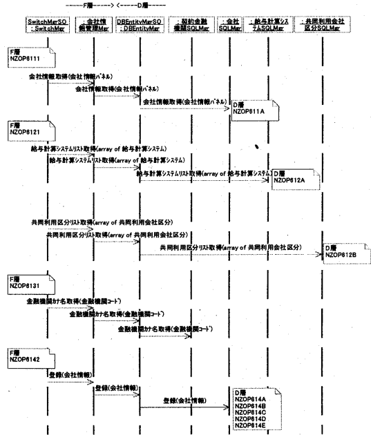
図 3-4 サーバー側シーケンス図
