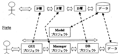
図 3-7 DORTIA から Forte へのマッピング
