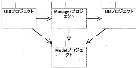
図 2-1 プロジェクトと可視性
