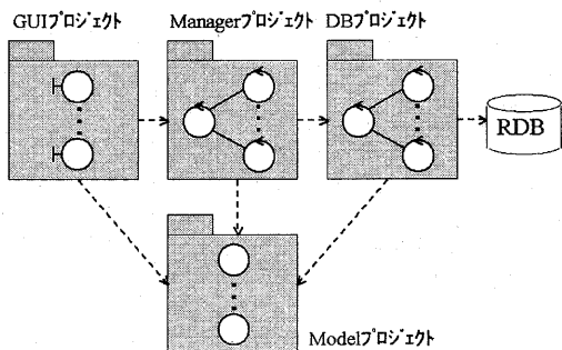
図 3-6 アーキテクチャ
