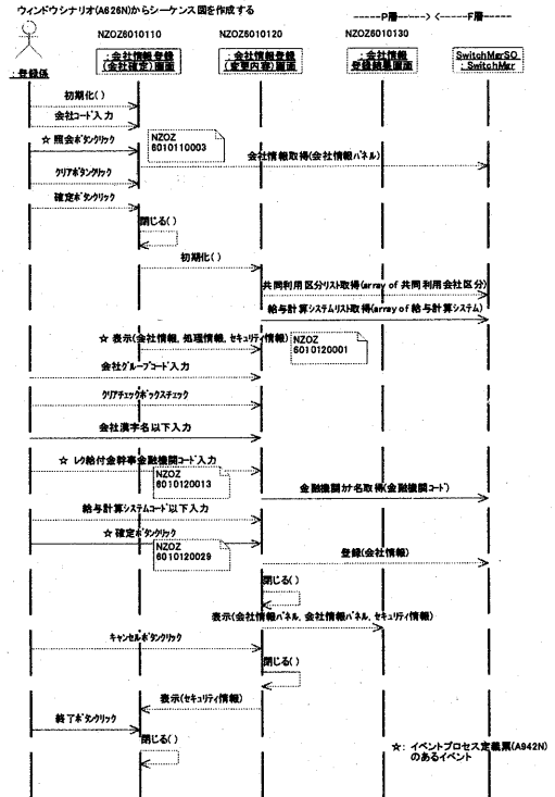
図 3-1 GUI 側シーケンス図
