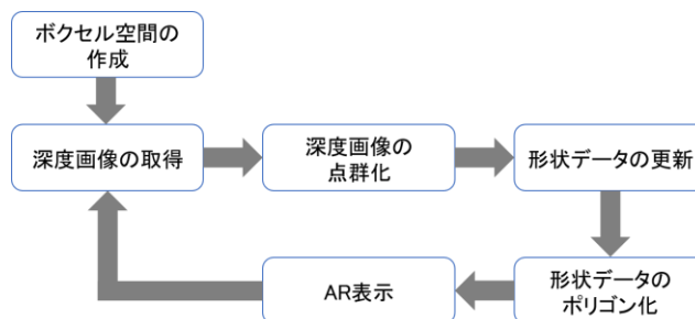
図2 システムの処理の流れ
