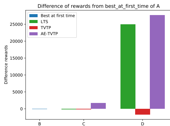
図4 Aグループを基準とした累積報酬の差の比較
