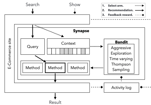
図 1 提案システムの処理フロー
