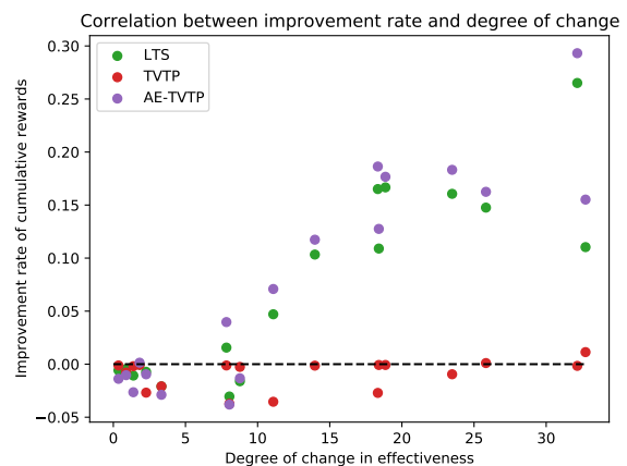
図5 推薦手法の有効性の変動度合いと累積報酬の改善率の相関
