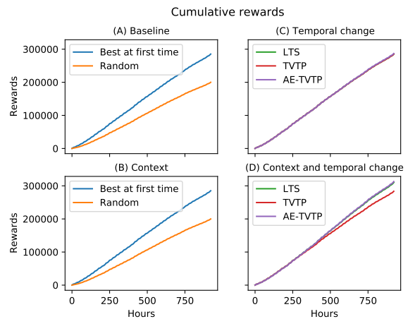
図3 累積報酬のシミュレーション間比較
