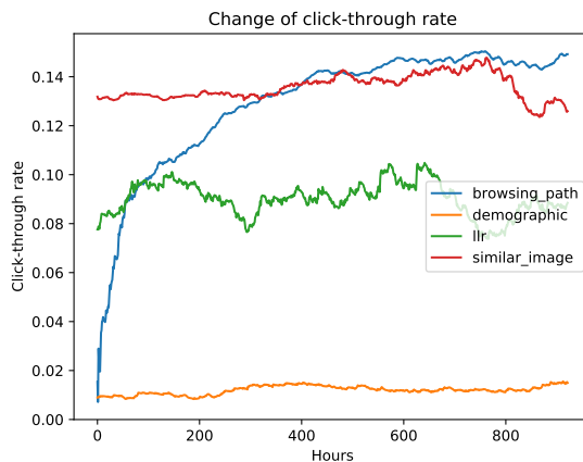
図2 推薦手法ごとのクリック率の推移
