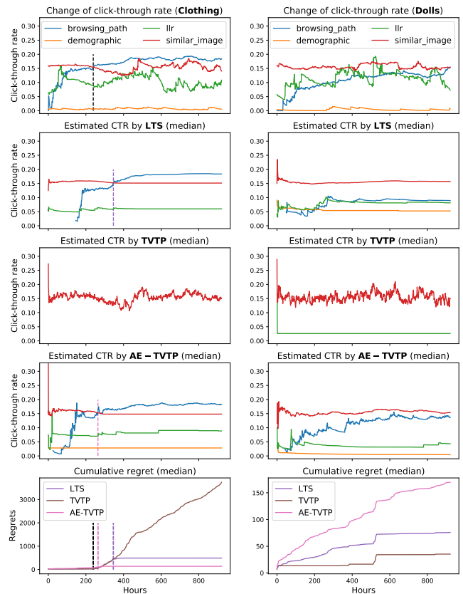
図6 Dグループの各シミュレーションにおけるクリック率、推定クリック率、累積リグレットの商品カテゴリ間比較。縦線はクリック率または推定クリック率が逆転した時点を示す。
