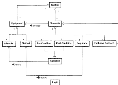
図1 システムのメタモデル
