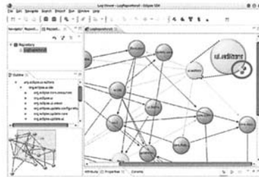
図 2 動的なプラグイン依存関係
