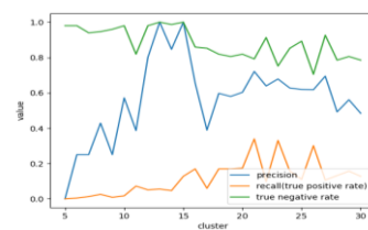
図3 最適なクラスタ数
