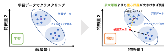
図1 クラスタリングによる異常検知
