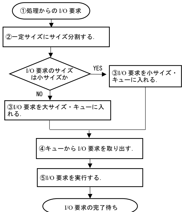
図 7 ディスク I/O 制御機構の処理流れ
