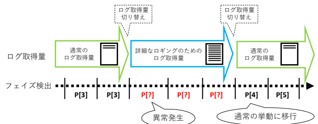
図 2 ログ取得量の動的制御
