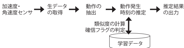
図 2 任意動作発生タイミング検出のアルゴリズム
