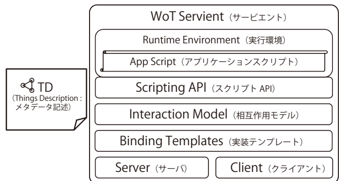
■ 図-2 WoT Servient Module
