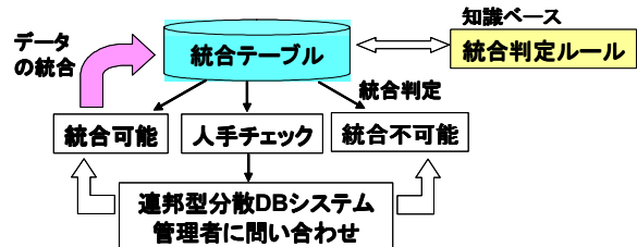
図 4: 個体統合処理の流れ
