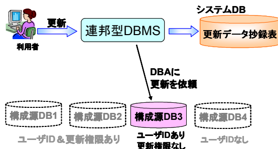
図 7：更新権限がない場合の更新処理
