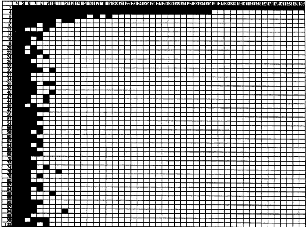
図 6 スпам長さ (横軸) と数 (縦軸) をパラメータとしたときの検出結果。黒いセルは検出可能、白いセルは検出不能
