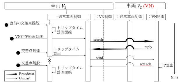
図 5 通常車両における、VN へのトリップタイム情報送信の流れ
