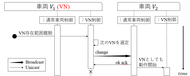
図 6 VN における、VN 存在範囲離脱時の VN の変更の流れ
