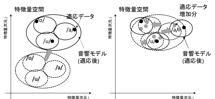
図 9 多段階話者適応における音響モデルの適応過程 (左: n 段階目の適応, 右: n+1 段階目の適応)
