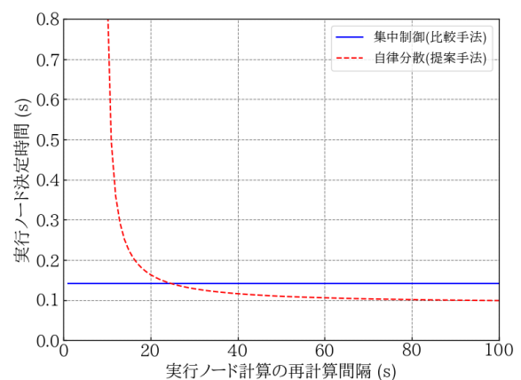
図 7 実験 2: エッジ環境数 100, エッジ環境あたりのノード数が 20 の場合の実行ノード決定時間
