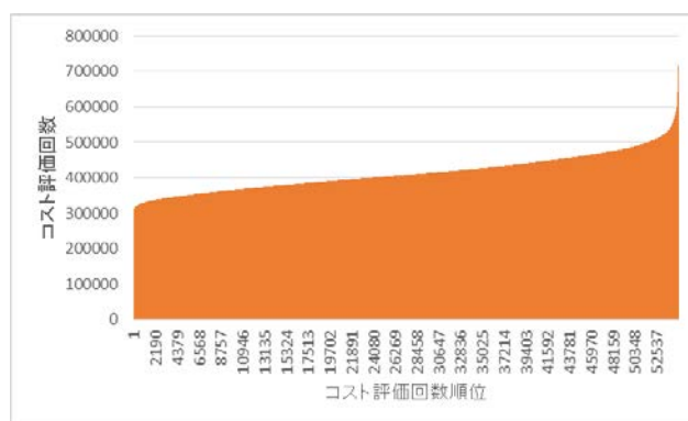
図4 条里制形状ネットワークにおけるコスト評価回数順位
