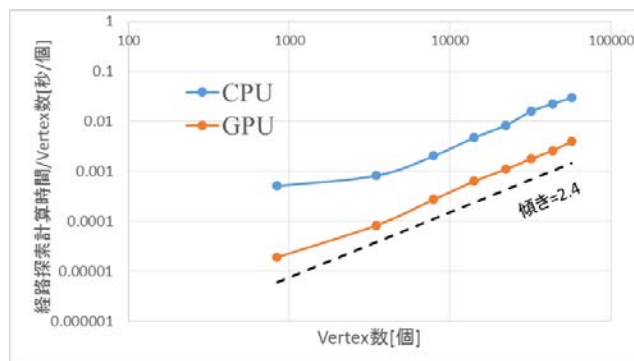
図3 経路探索計算時間のネットワーク規模依存性
