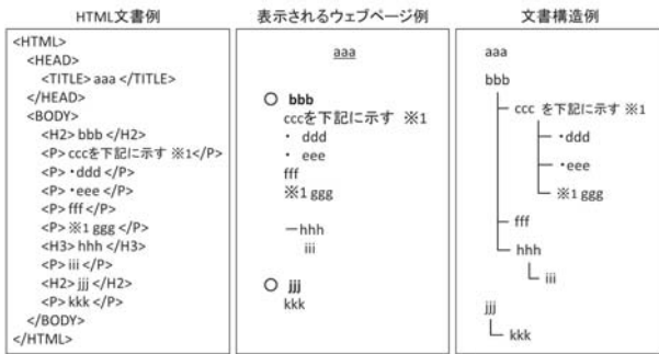
図 1 HTML 文書と文書構造の例
