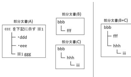
図 2 部分文書例
