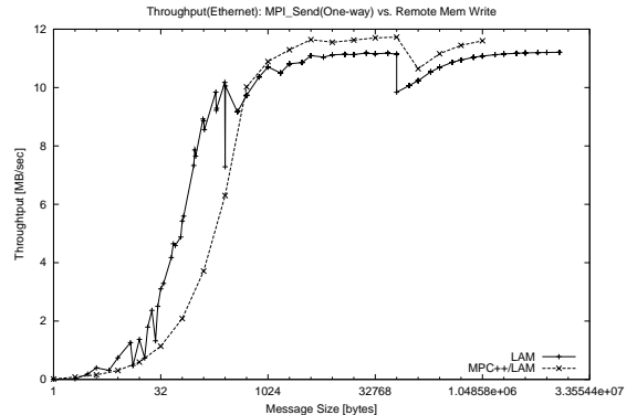
図 5 バンド幅 ( Ethernet ): LAM vs. MPC++/LAM Fig. 5 Throughput ( Ethernet ): LAM vs. MPC++/LAM.
