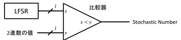
図 1 Stochastic Number の生成
