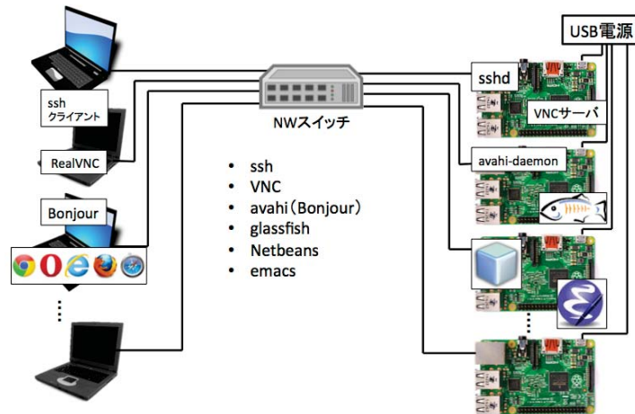
図 1 用意した演習環境.
