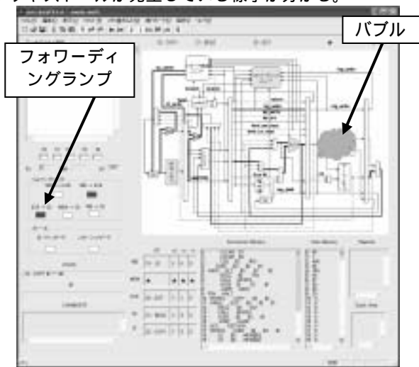
図 2：パイプライン選択時の実行画面
