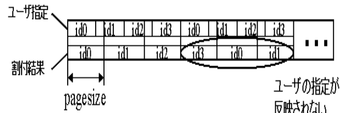
図2 JIAJIA の割付方式
