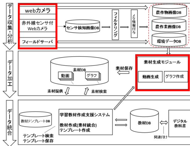
図 1.教材作成支援システム構成
